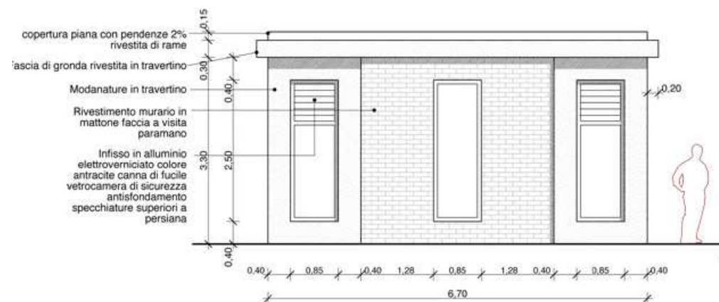
FRONTE LATERALE verso RAMPA CARRABILE
