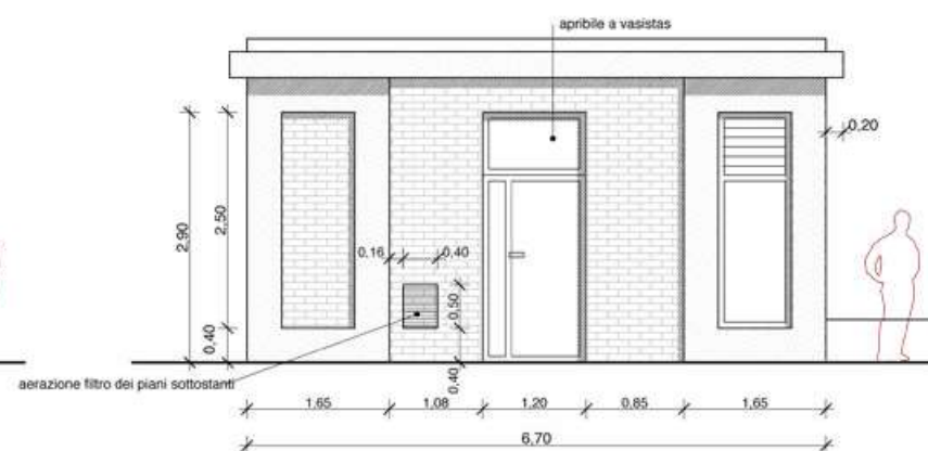
FRONTE LATERALE INGRESSO PEDONALE
