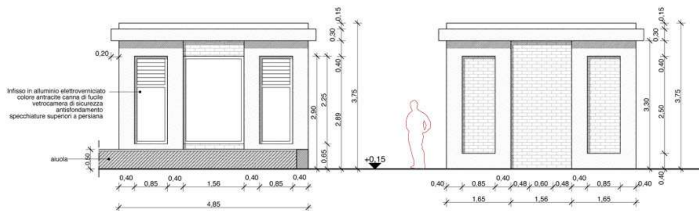
FRONTE verso AIUOLA RIALZATA
